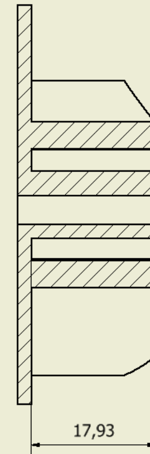
A-A ( 2 : 1 )
